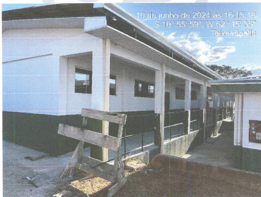
Figura 6: Esquadrias e guarda corpo instalados;
