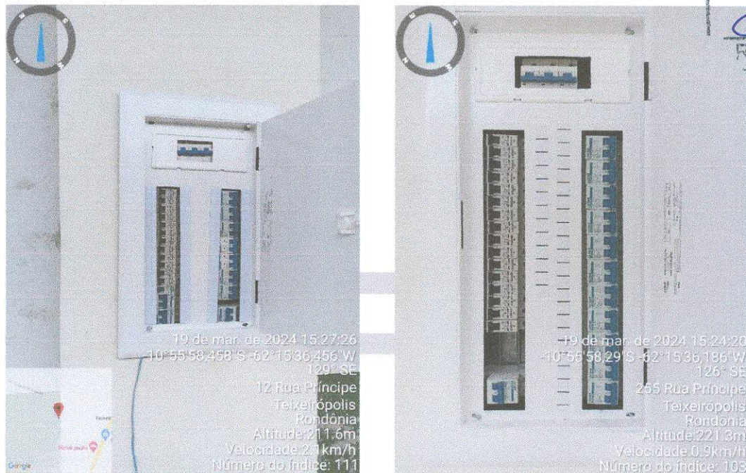
Figura 1: Quadros elétricos;
