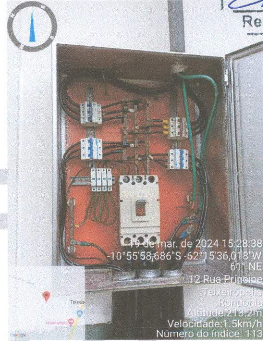
Figura 3: Quadros elétricos;
