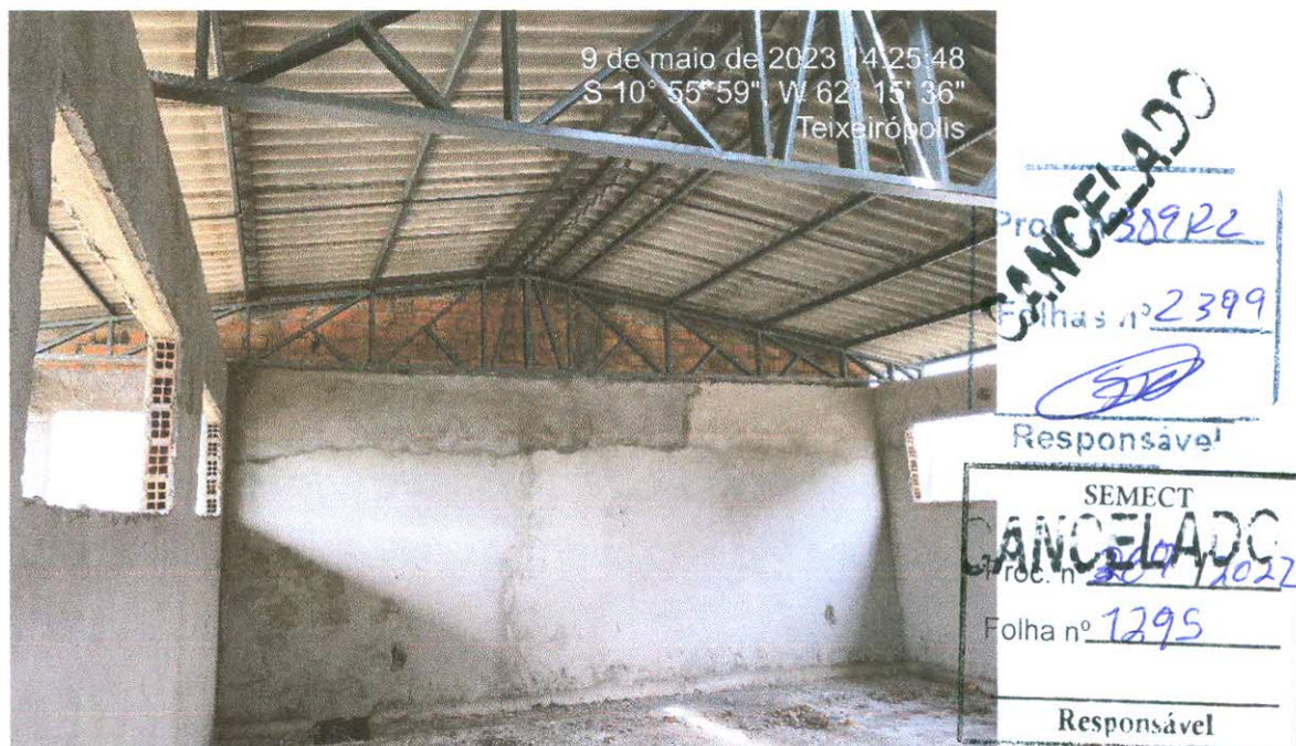
Figura 5: Telhamento com telha fibrocimento 6mm;
