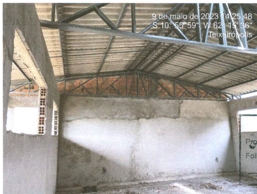
Figura 5: Telhamento com telha fibrocimento 6mm;
