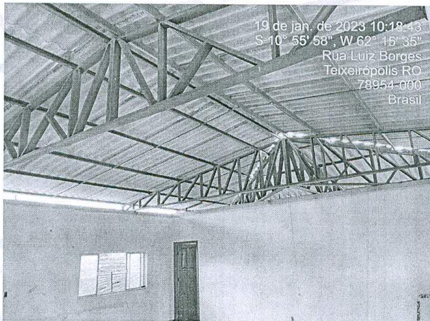
Figura 3: Telhamento com telha fibrocimento;
