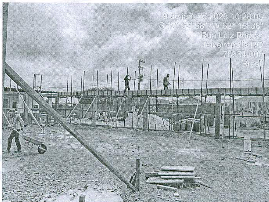
Figura 8: Pilares concretados e forma de viga respaldo sendo montada na área do pátio;
