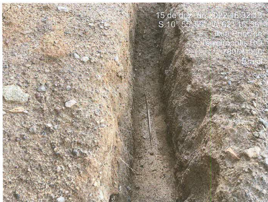
Figura 6: Cordoalha de cobre nu 50mm instalada;
